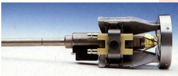
Selvrensende brænderhoved
