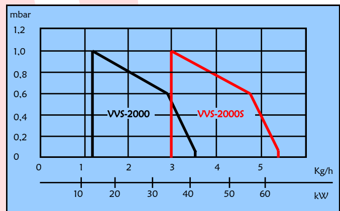
Kapacitetsdiagram
