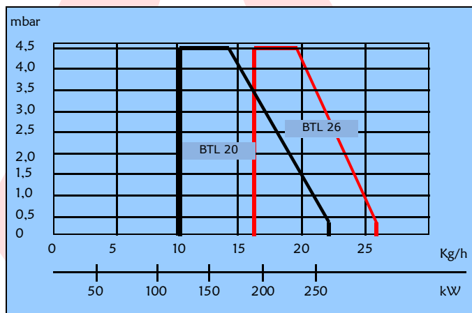
Kapacitetsdiagram
