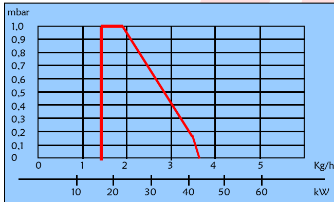
Kapacitetsdiagram
